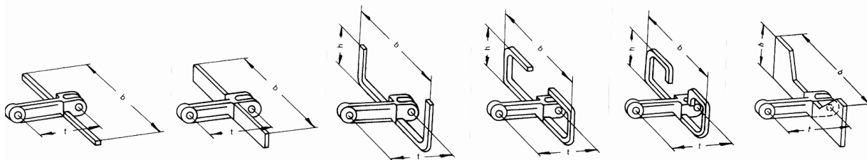
T - Kettenglied Square Bar Flight En Barre Tipo T
